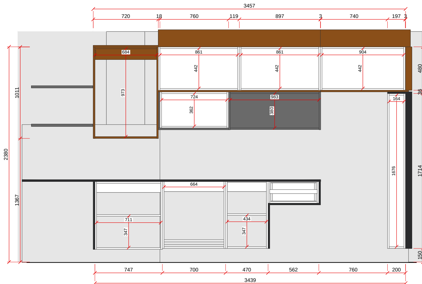
VISTA A - ESC. 1:25
