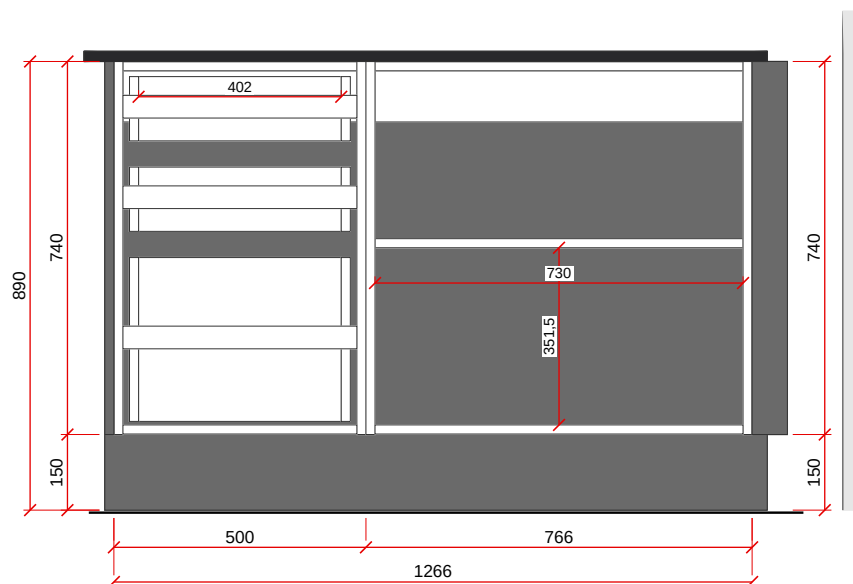
VISTA B - ESC. 1:15
